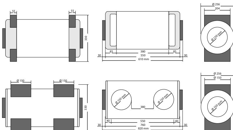
Joonis 4. Seadme PRANA-250 mõõdud.
