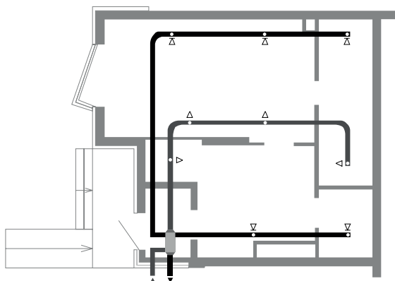
Joonis 7. PRANA-250 paigalduse näide
