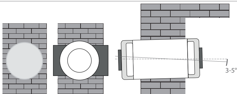
Joonis 8. Seadme paigaldus välisseina.
